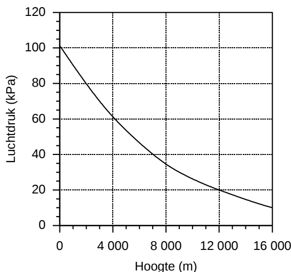
Figuur 2.20-3. Gemiddelde luchtdruk tegen de hoogte boven het aardoppervlak. Voorbeeld van een kromme grafiek.
