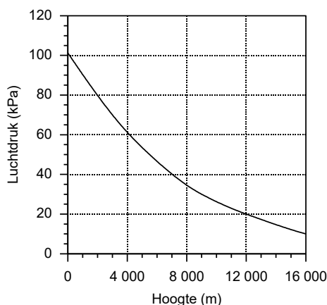
Figuur 2.14-1. Grafiek van luchtdruk in kPa tegen hoogte in m.
