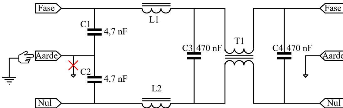
Figuur 17.4-4. Netfilter. Rood kruis: ontbrekende aarding in het stopcontact. Het gearde handje stelt verbinding met aarde via menselijke aanraking voor.
