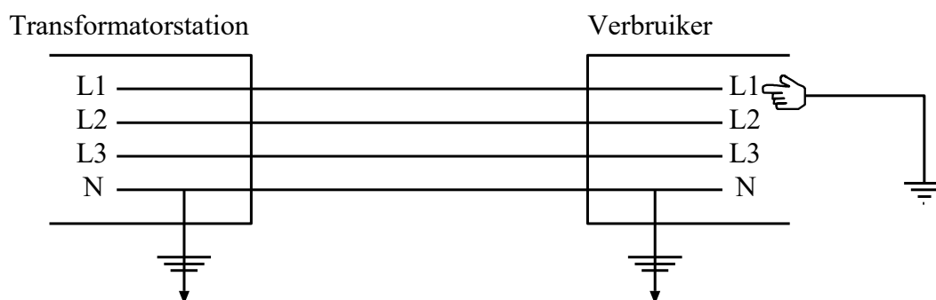
Figuur 17.4-1. Huisaansluiting. N staat voor Nulleiding, L voor faseLeiding 1-3.
