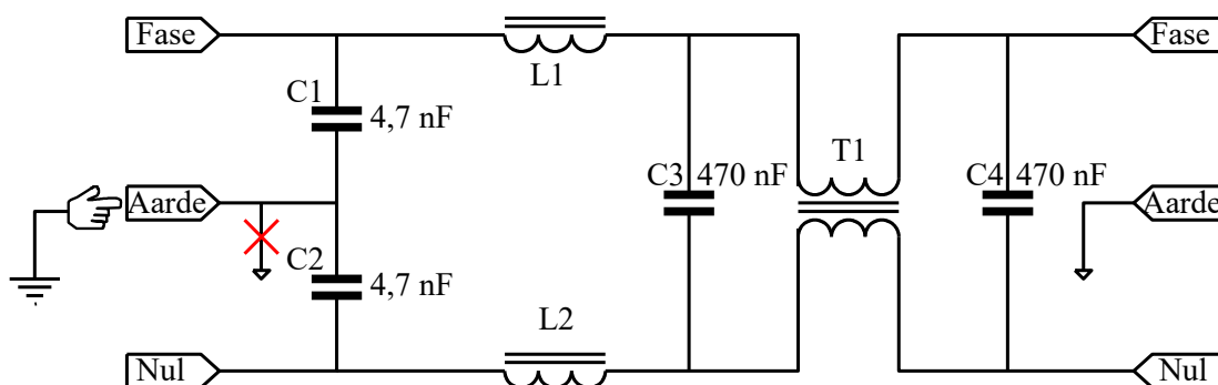
Figuur 17.4-4. Netfilter. Rood kruis: ontbrekende aarding in het stopcontact.
