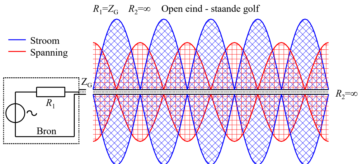
Figuur 14.3-31. Staande golven in een transmissielijn met open uiteinde. Op het uiteinde is de stroomgolf 0 en de spanninggolf maximaal.
