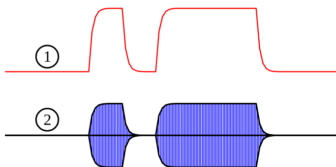
Figuur 12.2-11. Signaalsvorm bij CW met filtering. (1) bron; (2) gemoduleerd signaal.
