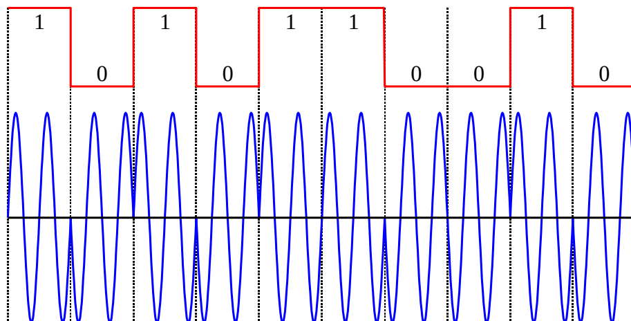
Figuur 12.3-3. Voorbeeld van BPSK. Een 1 begint op 0^\circ en een 0 op 180^\circ ( \pi ). Het aantal sinusperiodes per bit is groter dan in de tekening, maar voor de duidelijkheid van de figuur is dat aantal klein gehouden.
