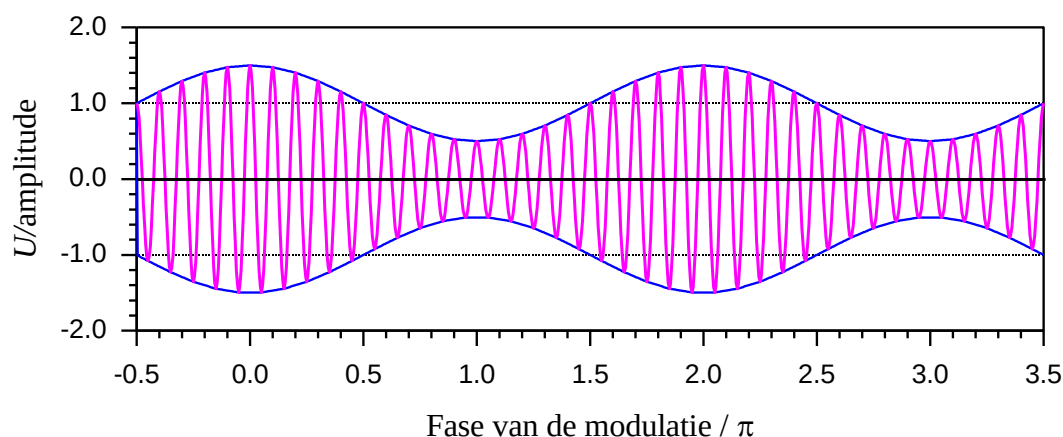
Figuur 12.2-3. AM-sigitaal als in Figuur 12.2-2, maar met AF-sigitaal met amplitude die de helft is van dat in Figuur 12.2-2,
