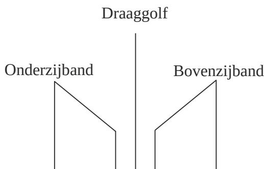
Figuur 12.2-5. Gestileerd frequentiespectrum van een AM-signaal met audiomodulatie (VRZA-cursus 1999).
