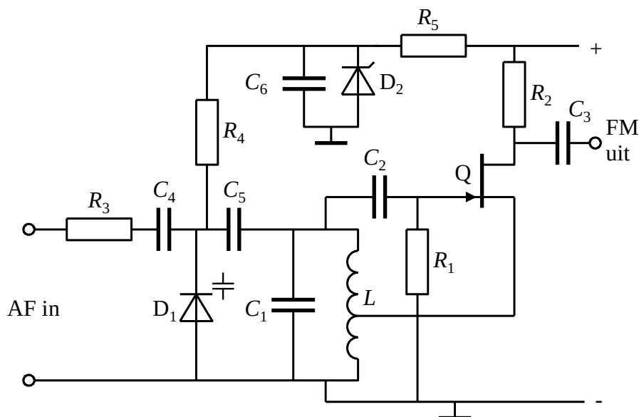
Figuur 12.4-17. FM met behulp van een varicap in een Hartley-oscillator.
