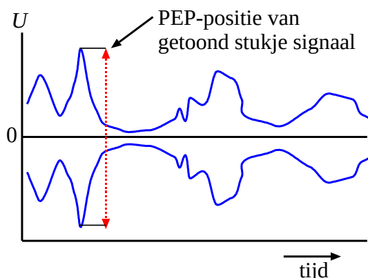
Figuur 12.2-7. Positie van PEP-punt in een stukje AM-modulatie dat wat meer “uit het leven gegrepen” is dan in vorige grafieken.
