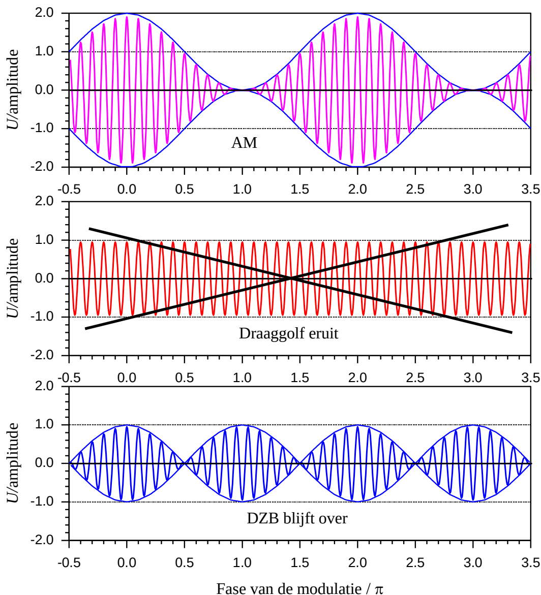
Figuur 12.2-8 Van AM naar DSB door verwijdering van de draaggolf.
